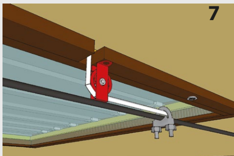
7 Colocación de la polea
