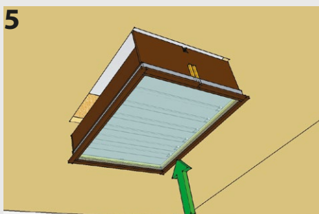
5 Colocación del tragaluz (sellar detrás del reborde)
