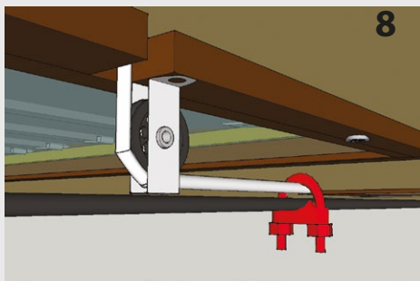
8 Fije la cuerda y el cable de tracción con la abrazadera de cable
