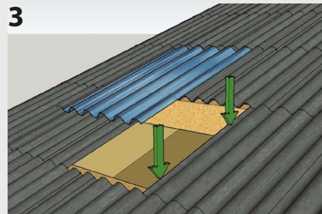
3 Coloque la chapa ondulada de luz natural
