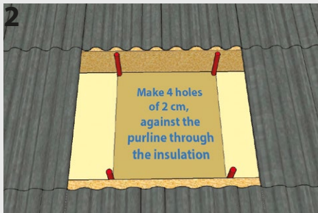
2 Haga 4 agujeros, 2 cm de diámetro a través del aislamiento
