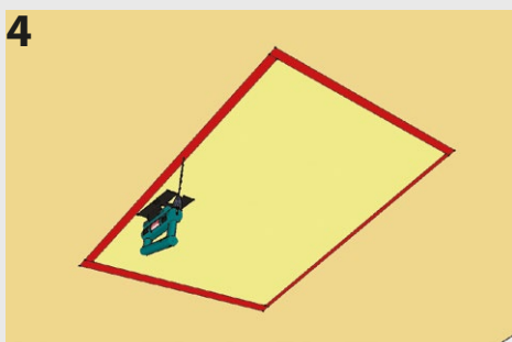
4 Corte el aislamiento
